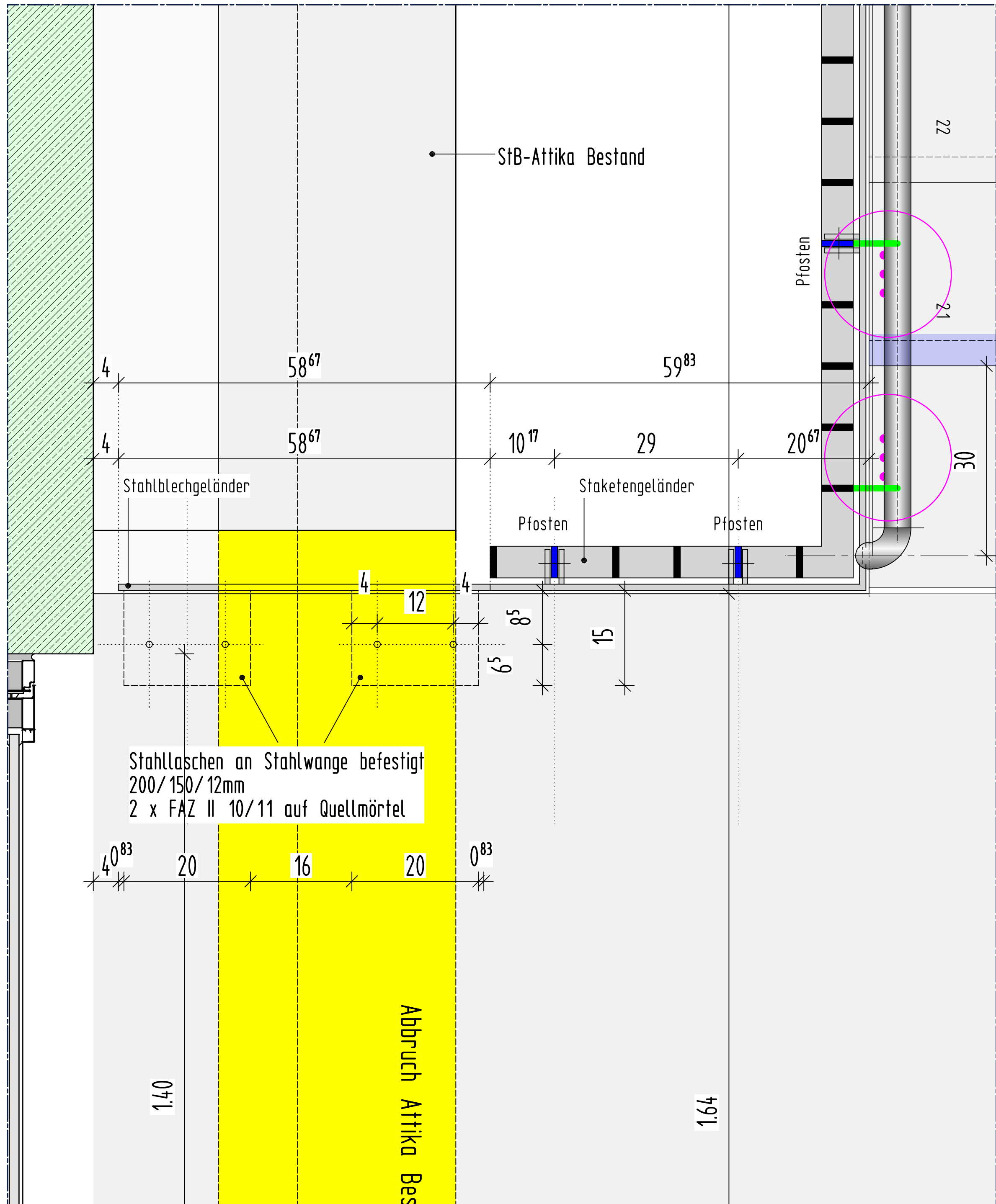
GRUNDRISSAUSSCHNITT 6-6 - Zwischenpodest 1.0G - M 1:5
