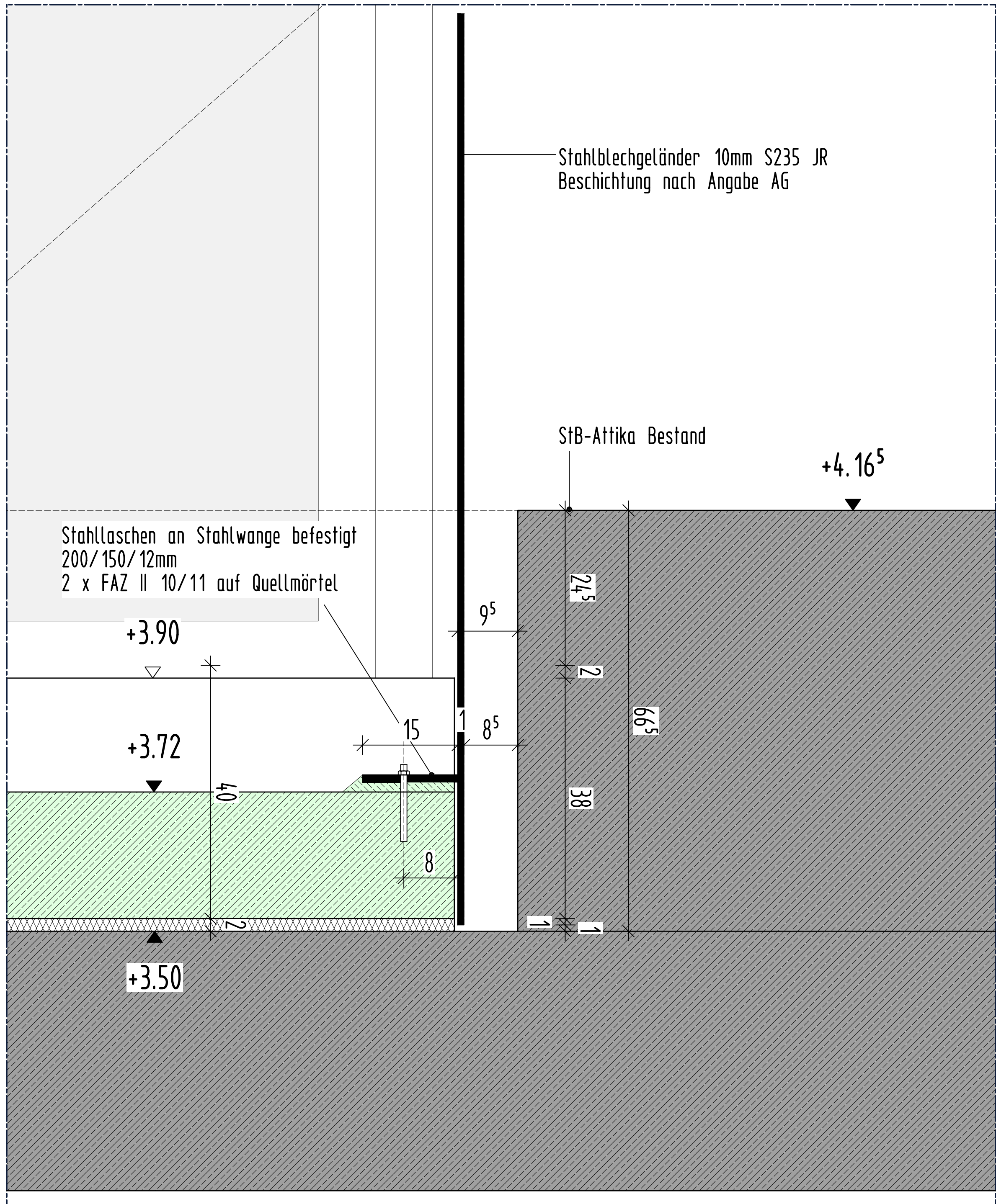
SCHNITT 5-5 - durch Stahlblechgeländer Hauptpodest 1.0G - M 1:5
