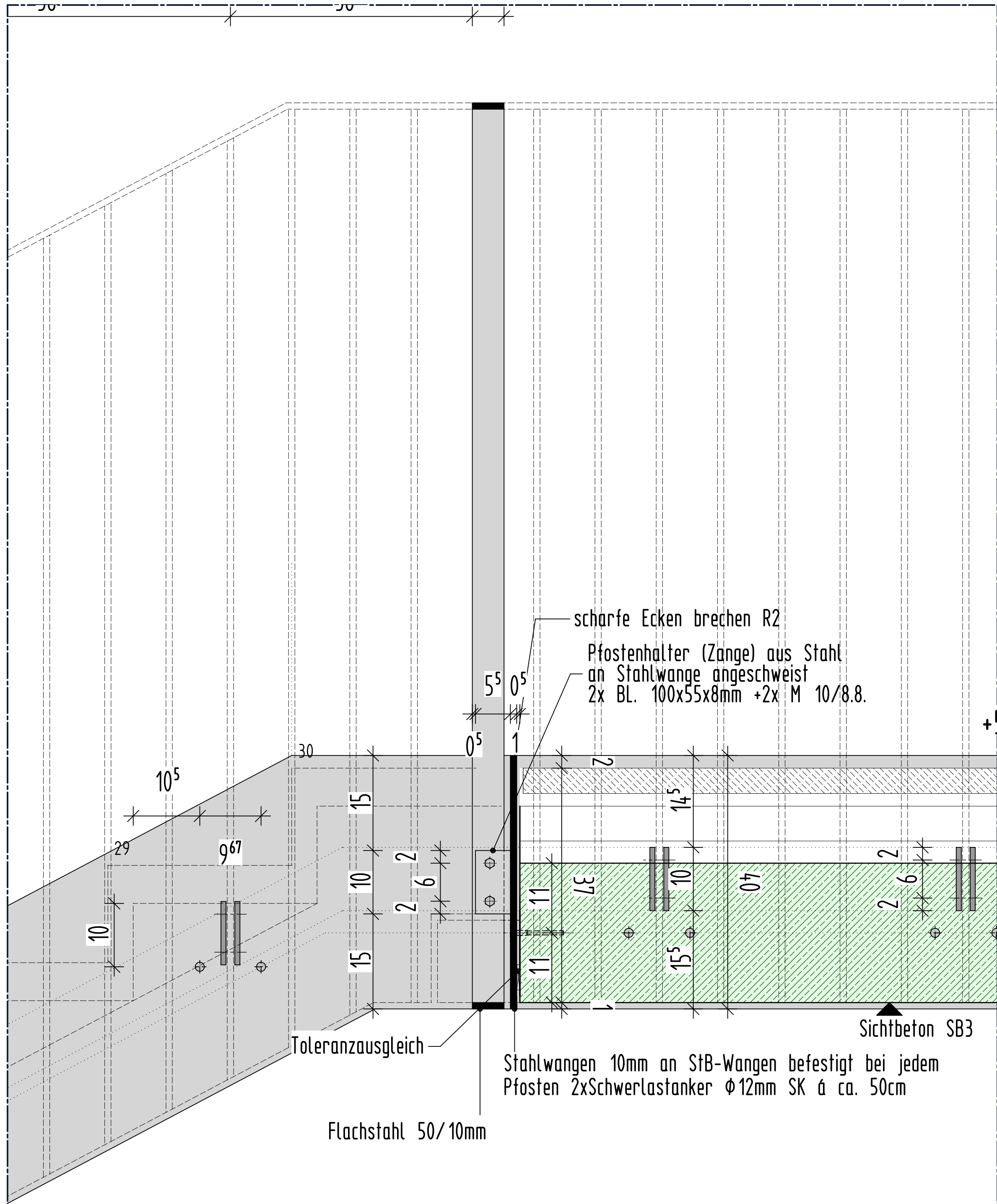
SCHNITT 8-8 - durch Treppenauge - M 1:5
