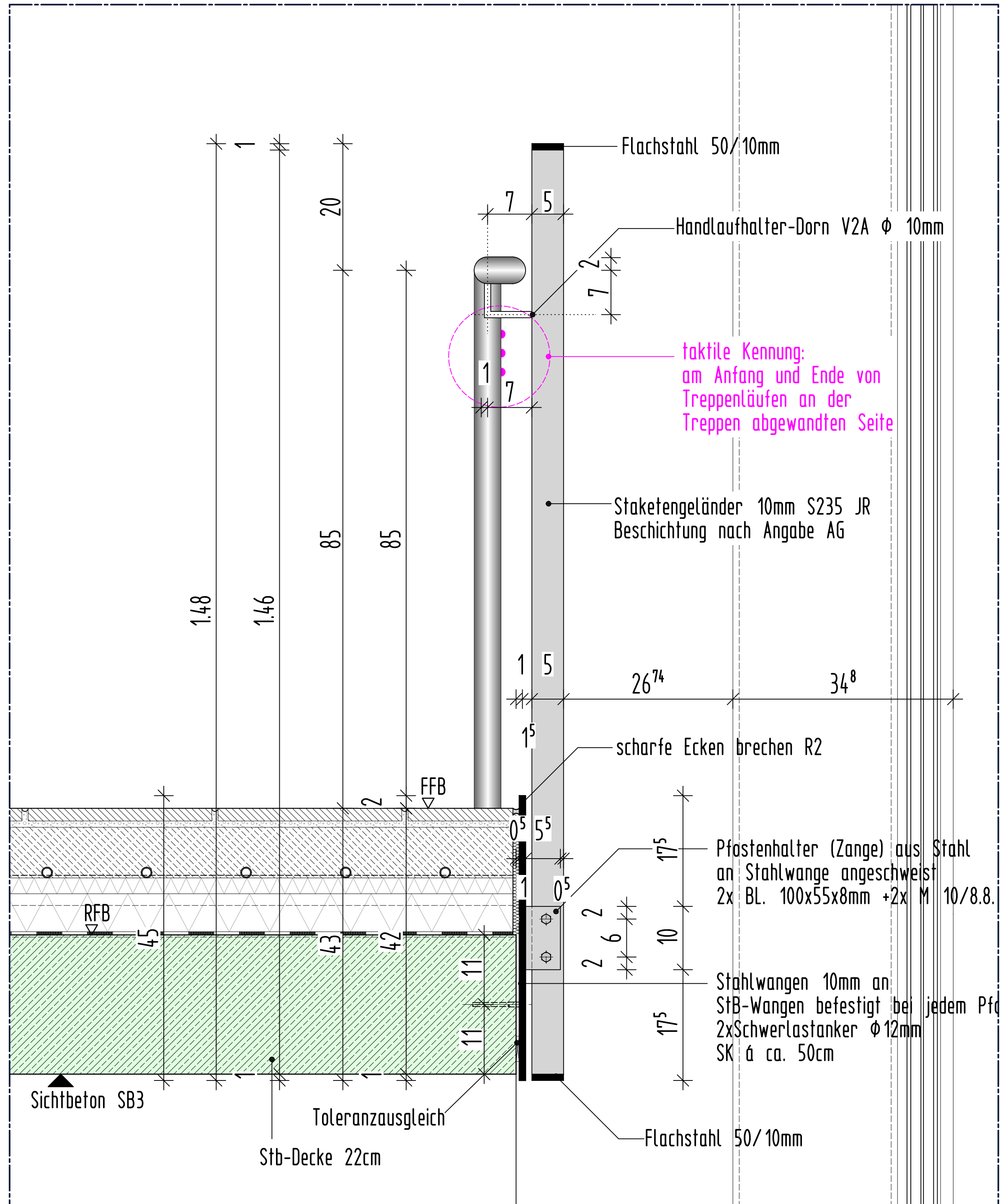
SCHNITT 4-4 - durch Staketengeländer an Hauptpodest - M 1:5
