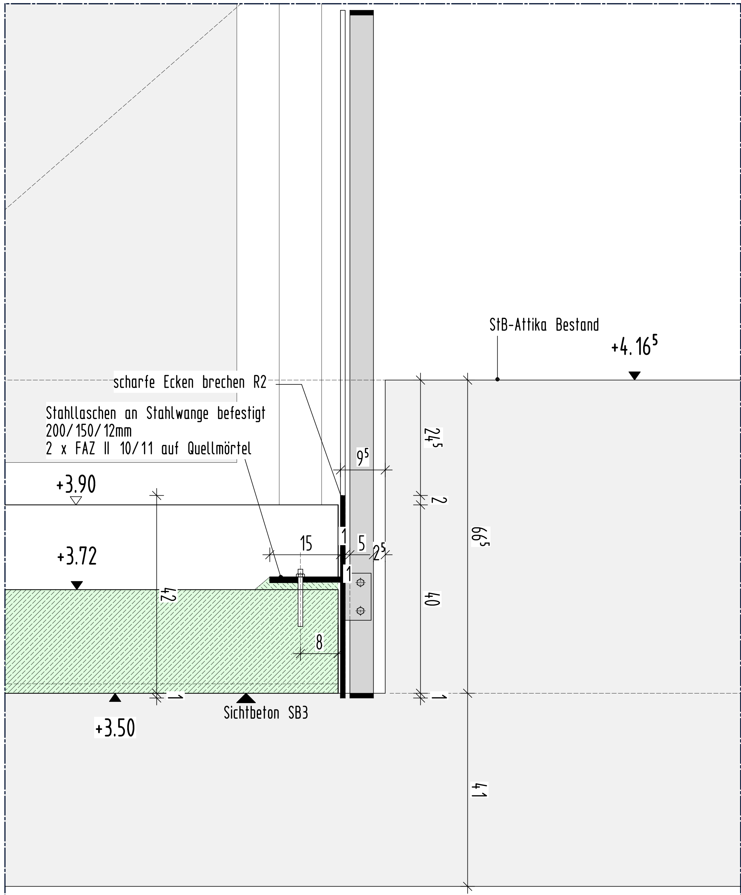
SCHNITT 7-7 - durch Staketengeländer Hauptpodest 1.0G - M 1:5
